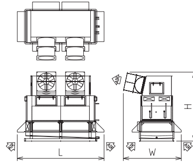
■ 寸法図：B型
